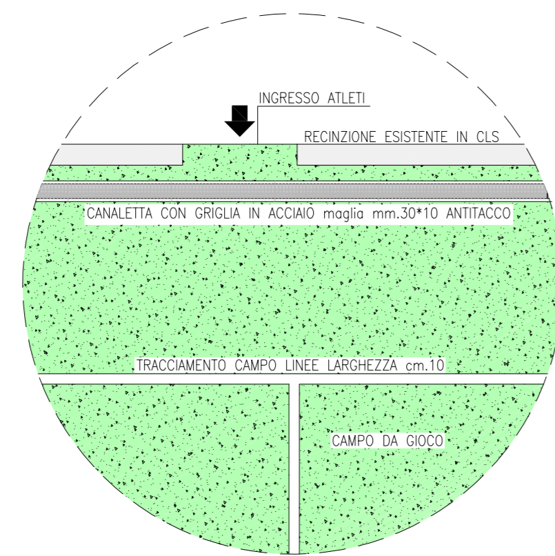
PARTICOLARE ESECUTIVO "P1" scala 1:50
